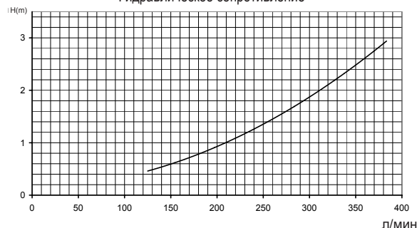
Гидравлическое сопротивление
