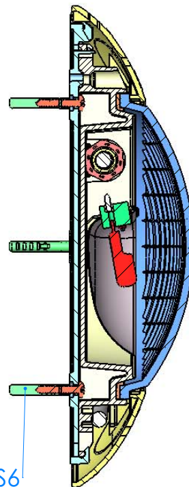
SECCIÓN A-A
